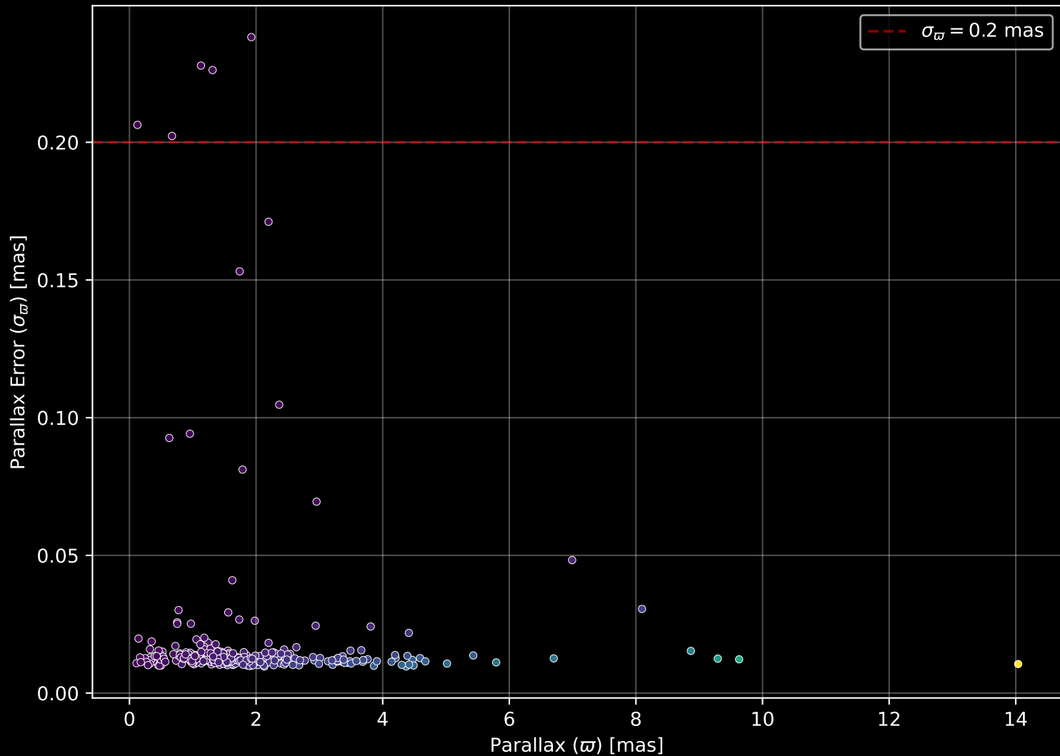
GALAH DR4 Field: [6930] Parallax Quality (n= 300)
