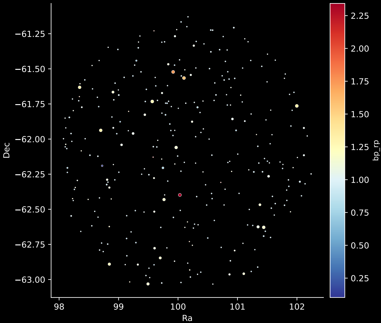
GALAH DR4 Field: [6930] Stars: 300
