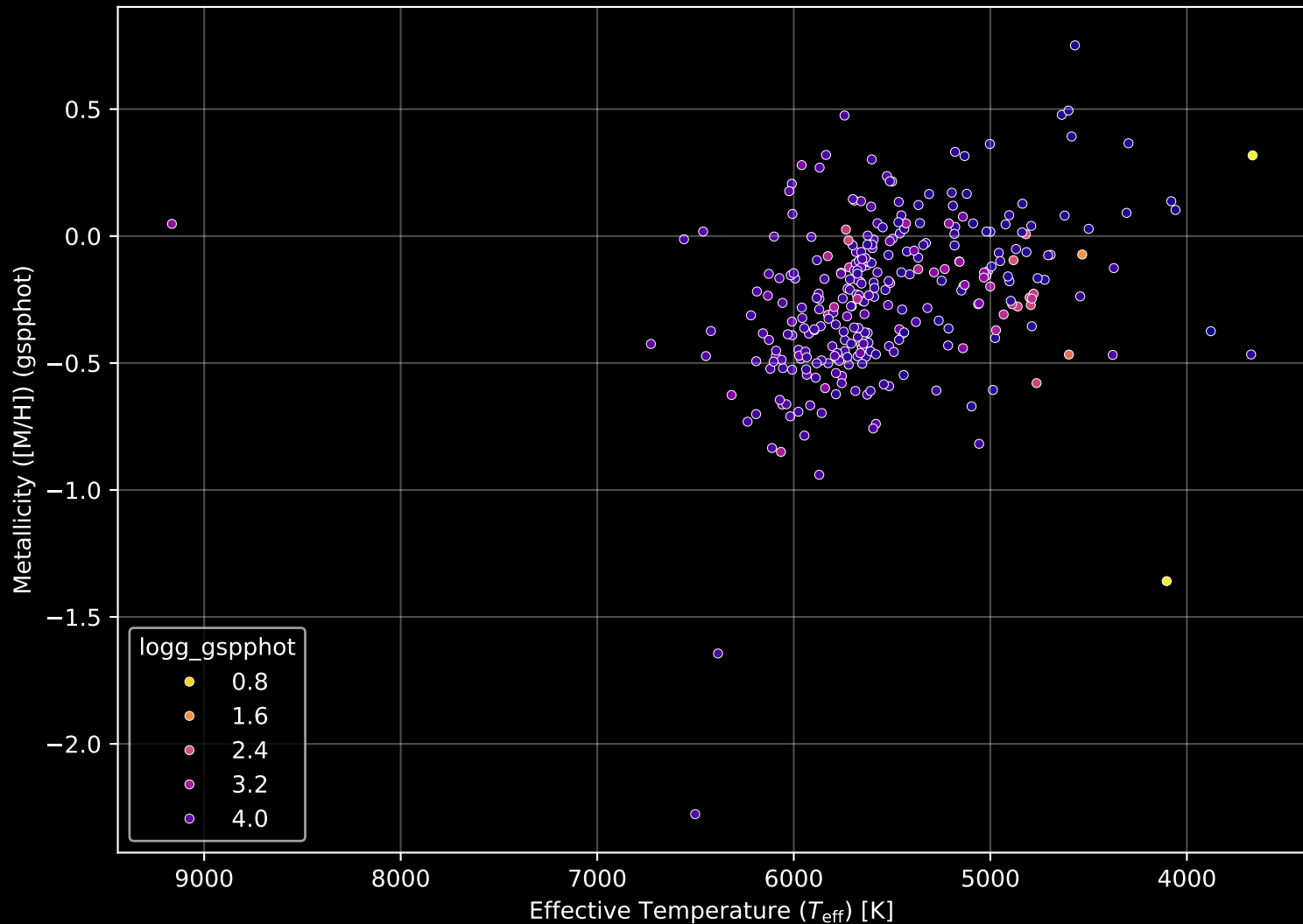
GALAH DR4 Field: [6930] Stellar Population Parameters (n= 300)
